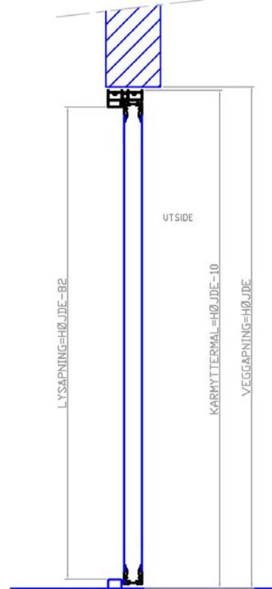
Vertikalseksjon
