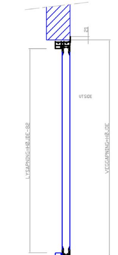
Vertikalseksjon
